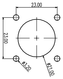
插座面板开孔图
