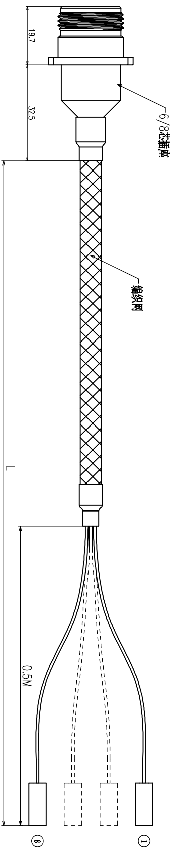
插座组件
