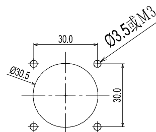
8Cores Socket (ZDC08S)
