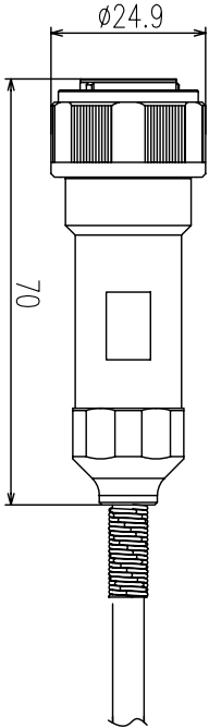
D38999 III PLUG ARINC 801
